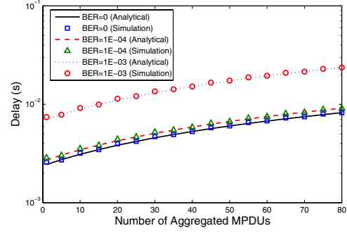
Fig. 8. Access Delay for A-MPDU.
